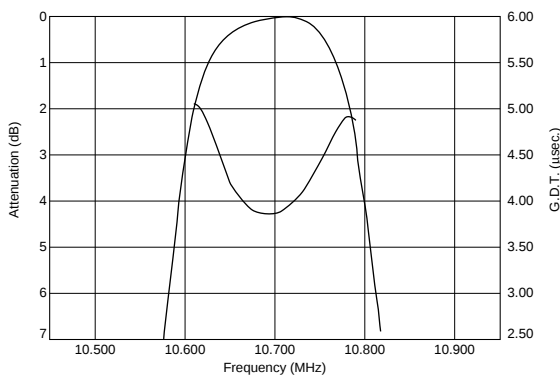
SFECV10M7HA00-R0
