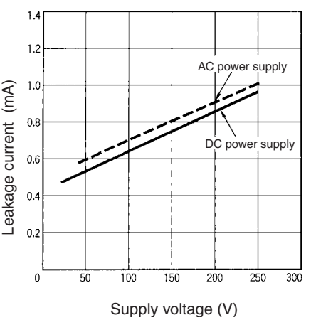
E2E-X□T1 DC/AC
