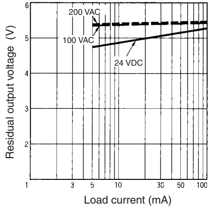
E2E-X□T1
