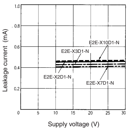
E2E-X□D□
