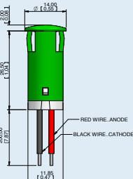
WIRES
