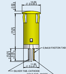
SOLDER LUG/FASTON
