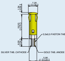
SOLDER LUG/FASTON
