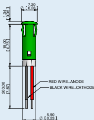
WIRES
