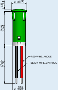
WIRES
