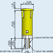
SOLDER LUG/FASTON
