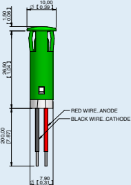
WIRES
