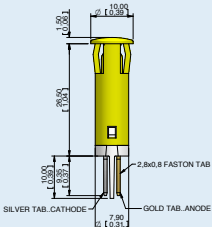
SOLDER LUG/FASTON
