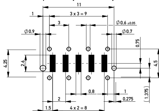
Leiterplatten-Layout / PCB-Layout
