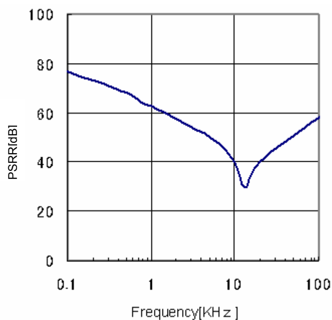
Fig.21 PSRR ( I_o=0 mA)
