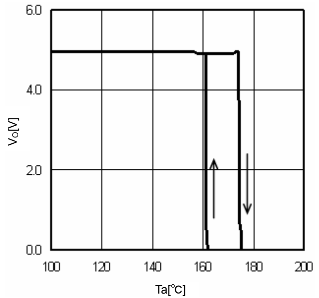
Fig.16 TSD ( I_O=0mA )
