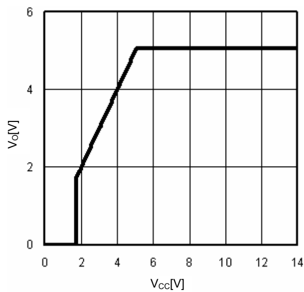
Fig.15 V_{CC}-V_O ( I_O=0mA )
