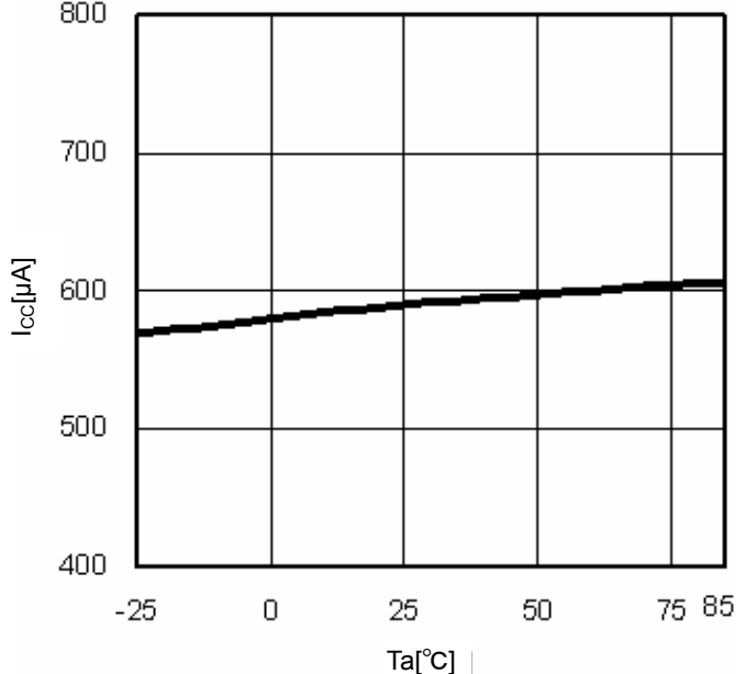
Fig.10 Ta-I CC
