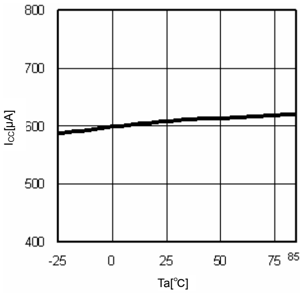
Fig.10 T_a-I_{CC}
