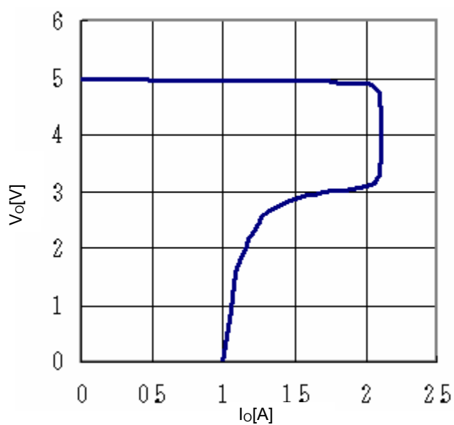
Fig.17 OCP
