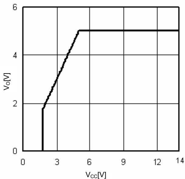
Fig.15 V_{CC}-V_O ( I_O=0\text{mA} )
