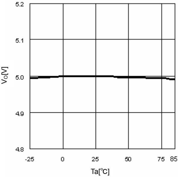
Fig.9 T_a-V_O ( I_o=0mA )
