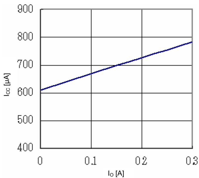
Fig.20 I_o - I_{cc}
