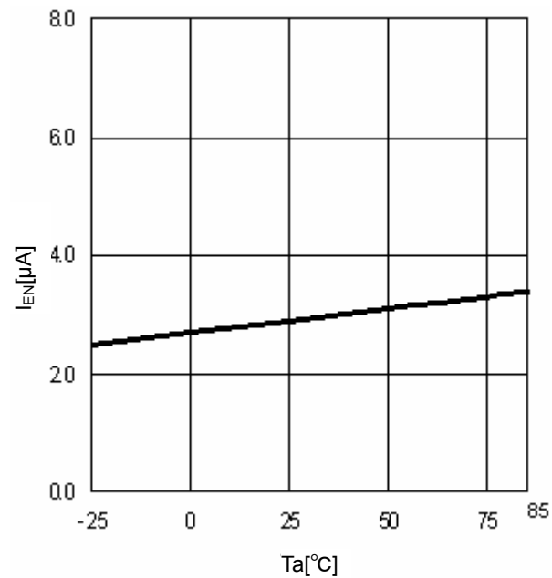
Fig.12 T_a - I_{EN}
