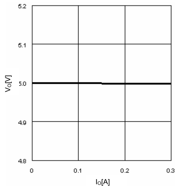
Fig.13 I_O - V_O
