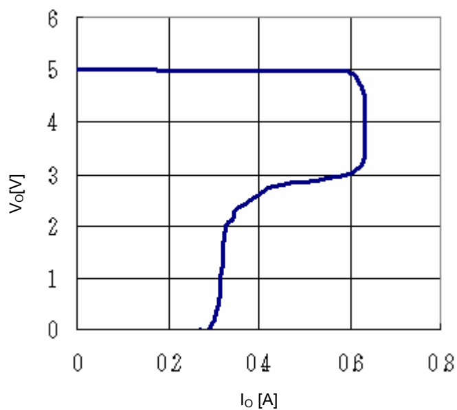
Fig. 17 OCP
