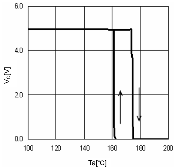
Fig. 16 TSD ( I_O=0\text{mA} )
