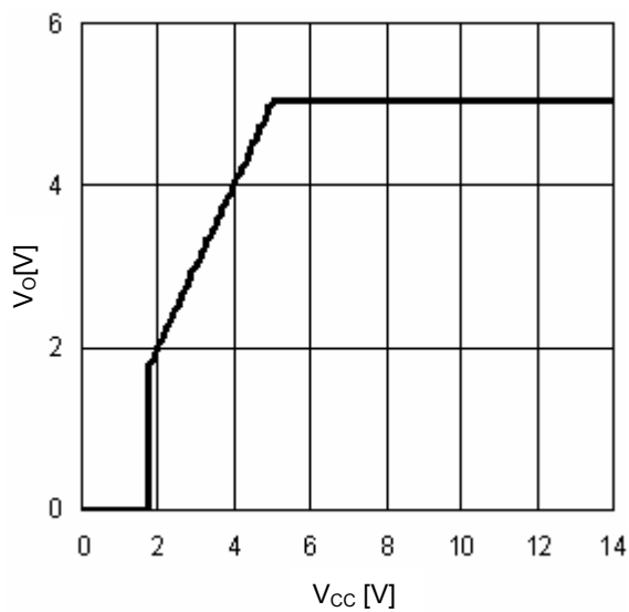
Fig. 15 V_{CC}-V_O ( I_O=0\text{mA} )
