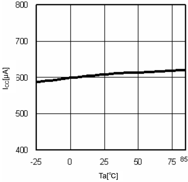
Fig.10 T_a-I_{cc}
