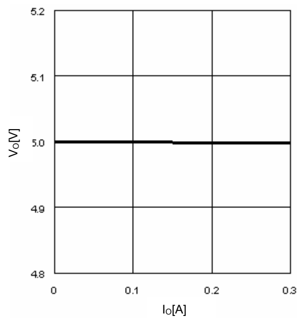
Fig.13 I_O - V_O
