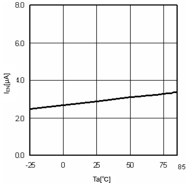
Fig.12 T_a - I_{EN}
