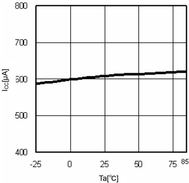
Fig.10 T_a-I_{cc}
