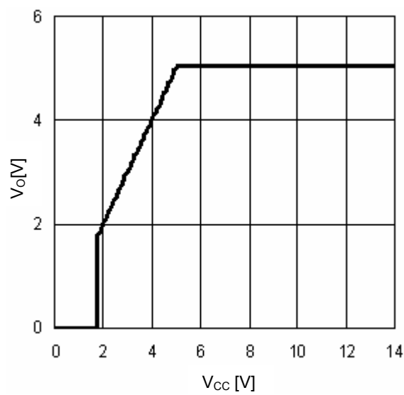
Fig.15 V CC -V O (I O =0mA)
