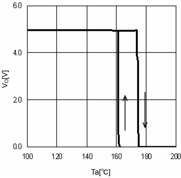
Fig.16 TSD (I O =0mA)
