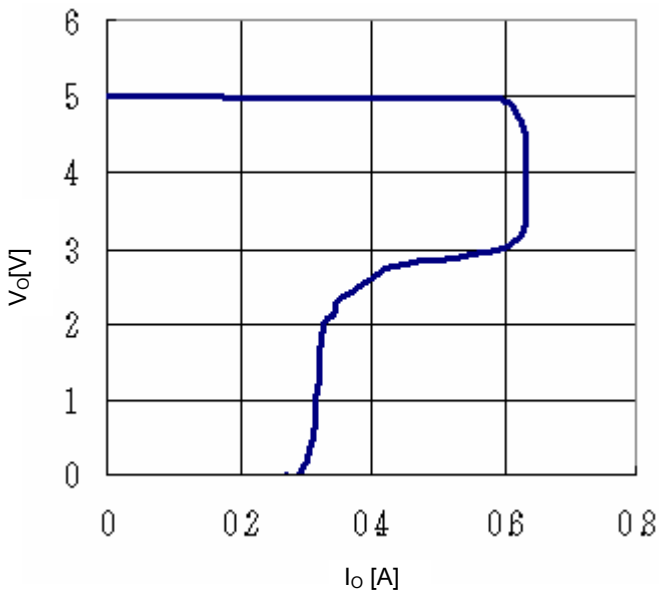
Fig.17 OCP
