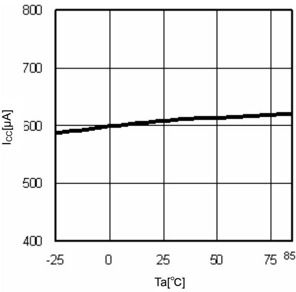
Fig.10 T_a-I_{cc}
