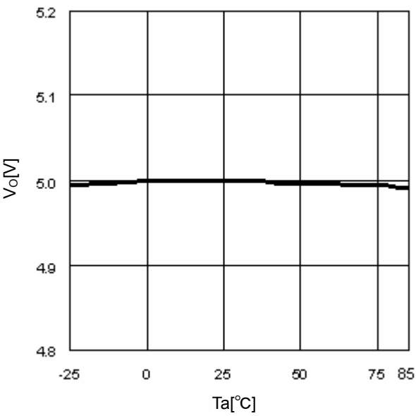
Fig.9 T_a-V_O ( I_O=0mA )
