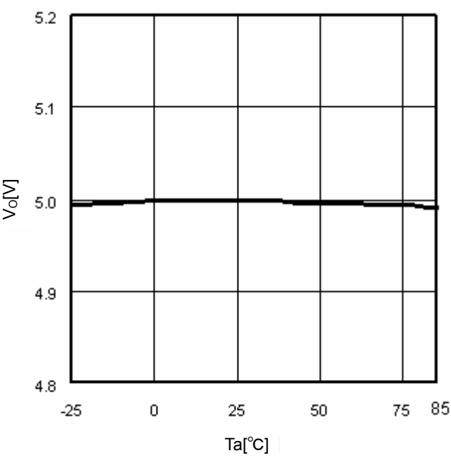
Fig.9 T_a - V_O ( I_o=0\text{mA} )
