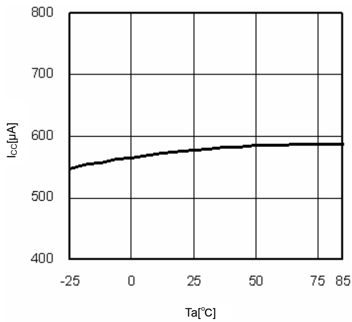
Fig.10 T_a - I_{CC}
