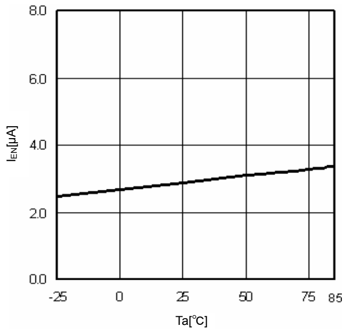
Fig.12 T_a - I_{EN}
