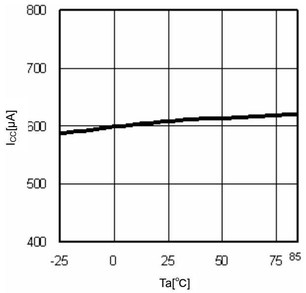
Fig.10 Ta-I CC
