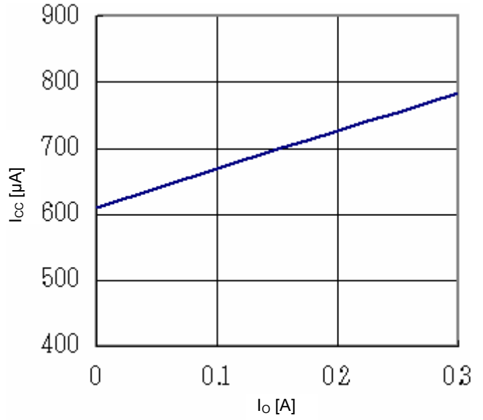
Fig.20 Io-Icc
