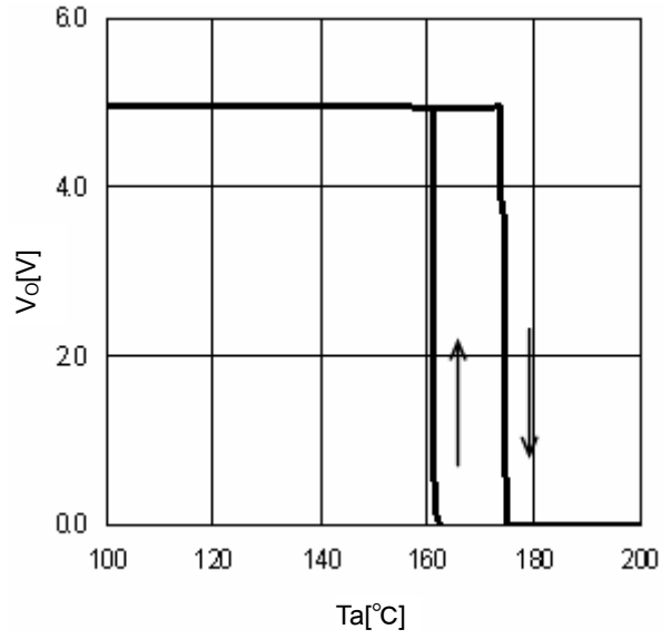
Fig.16 TSD ( I_o=0mA )
