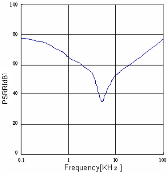
Fig.21 PSRR(Io=0mA)
