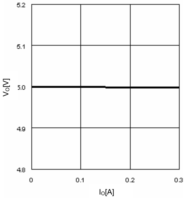
Fig.13 I O -V O
