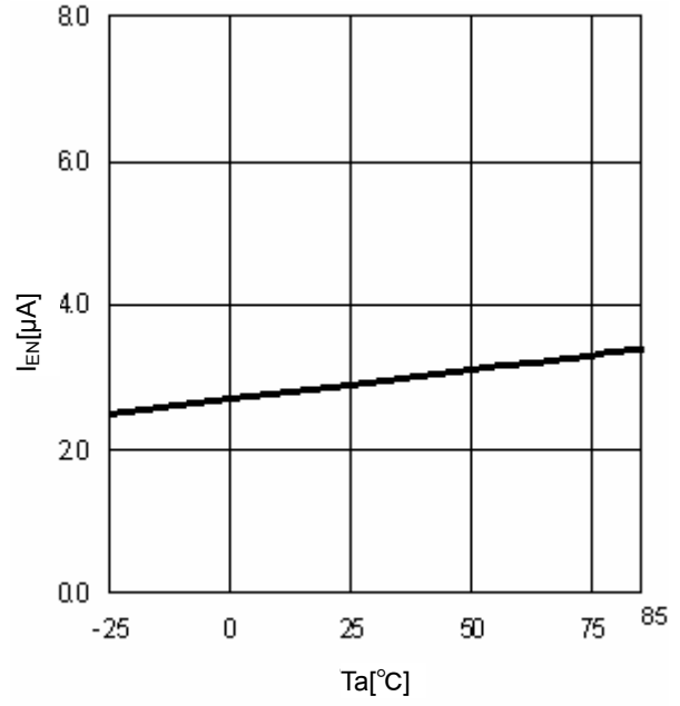
Fig.12 Ta-I EN
