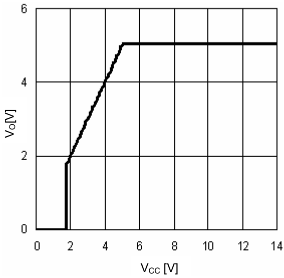
Fig.15 V_{CC}-V_o ( I_o=0mA )
