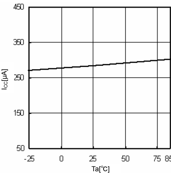
Fig.10 T_a-I_{cc}
