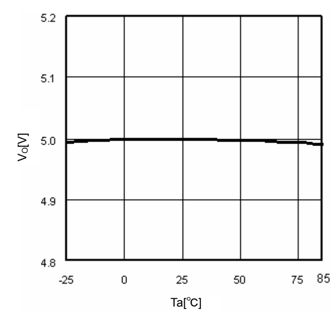
Fig.9 T_a-V_O ( I_O=0mA )
