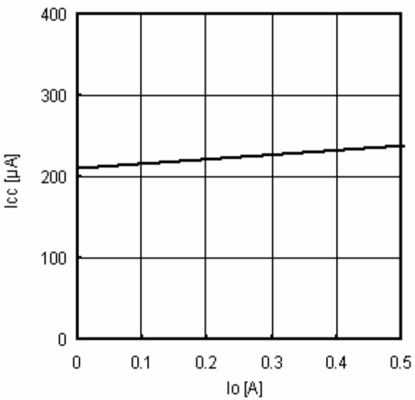
Fig.20 Io-Icc
