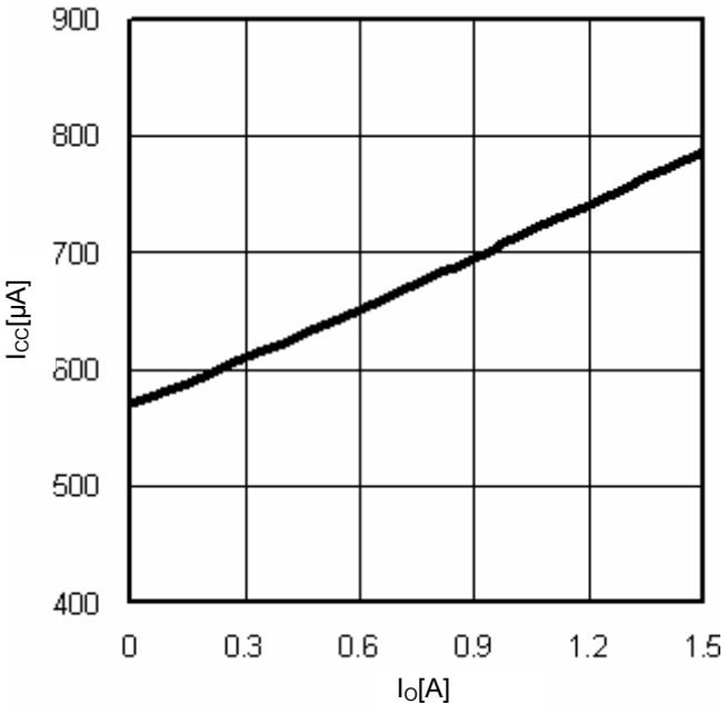
Fig.20 I_o - I_{cc}
