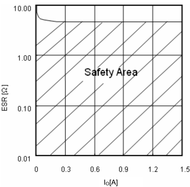
Fig.19 ESR condenser
