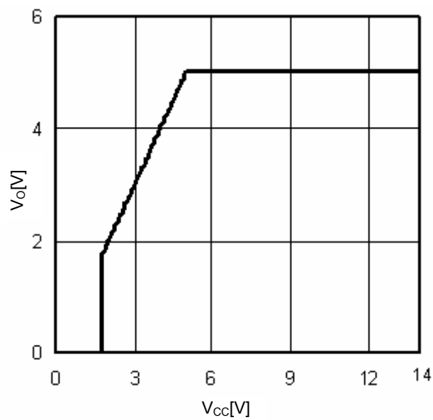
Fig.15 V_{cc}-V_o ( I_o=0mA )
