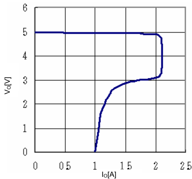
Fig.17 OCP
