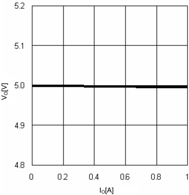
Fig.13 I_O - V_O
