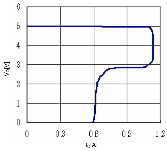
Fig.17 OCP
