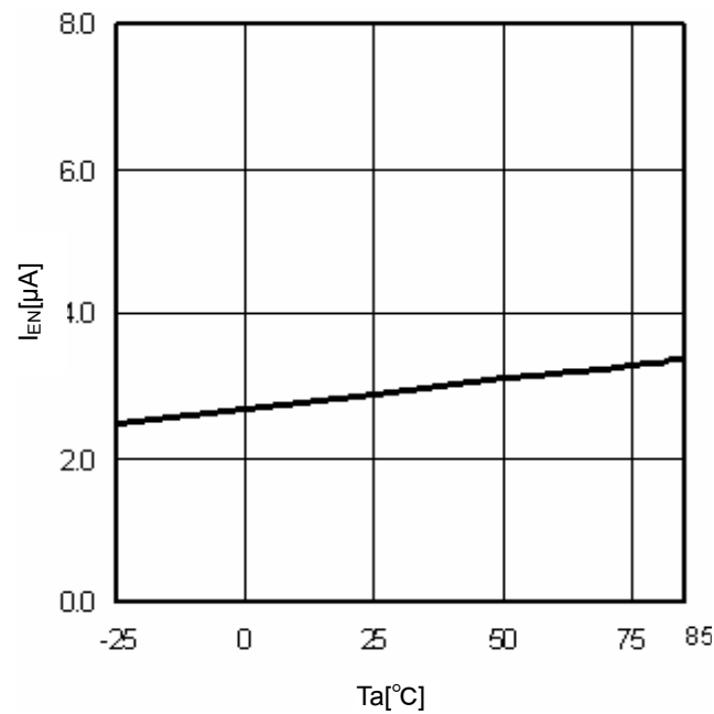
Fig.12 T_a - I_{EN}
