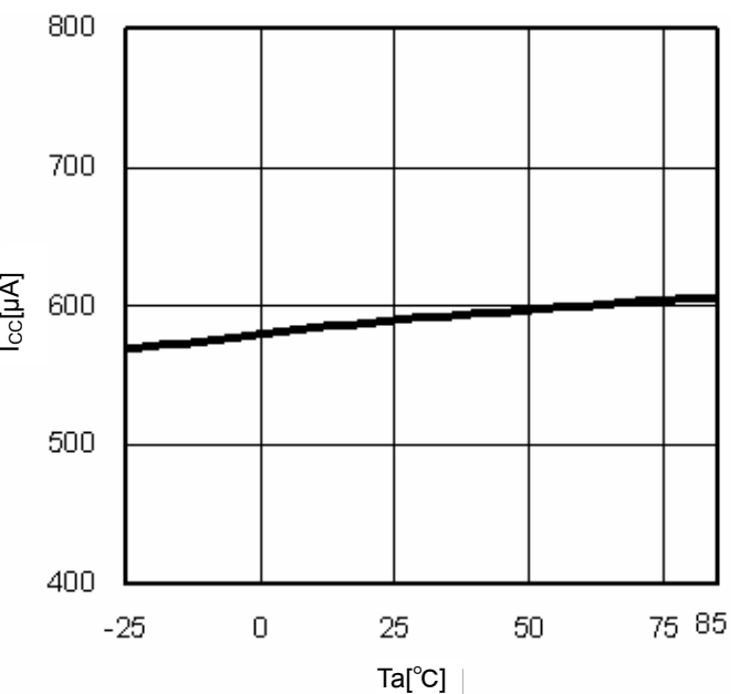
Fig.10 Ta-I CC
