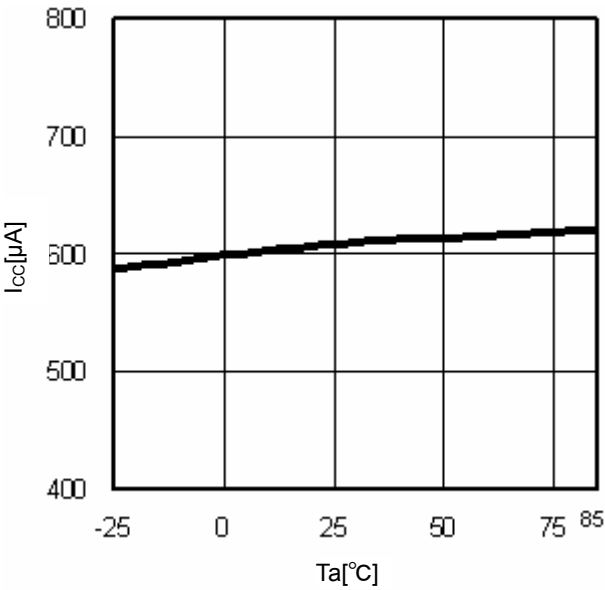
Fig.10 T_a - I_{cc}
