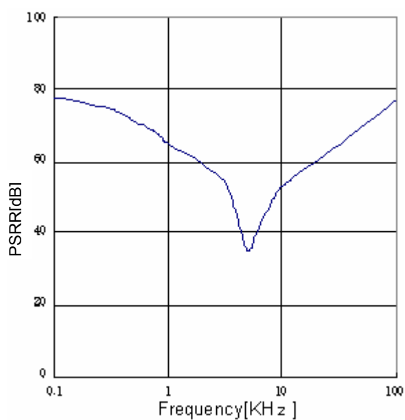
Fig.21 PSRR( I_o=0\text{mA} )
