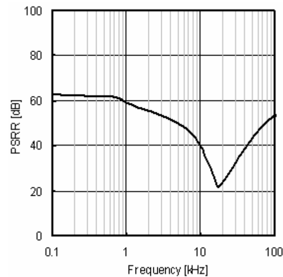
Fig.21 PSRR( I_o=0 mA)
