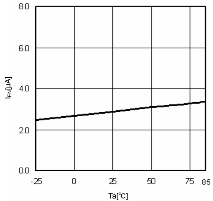
Fig.12 T_a - I_{EN}
