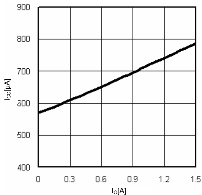
Fig.20 I_o - I_{cc}
