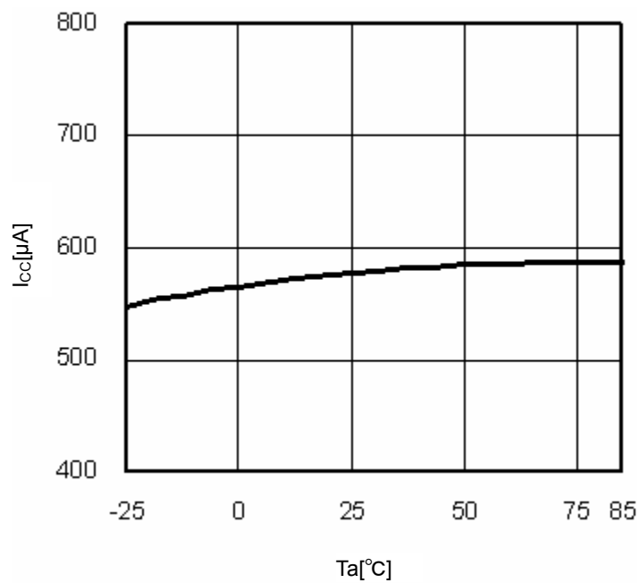
Fig.10 T_a-I_{cc}
