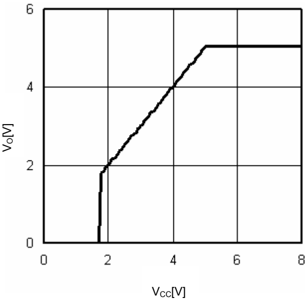
Fig.15 V_{cc}-V_o ( I_o=0mA )
