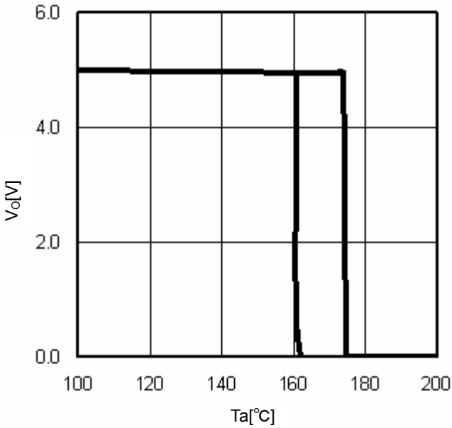
Fig.16 TSD ( I_o=0mA )
