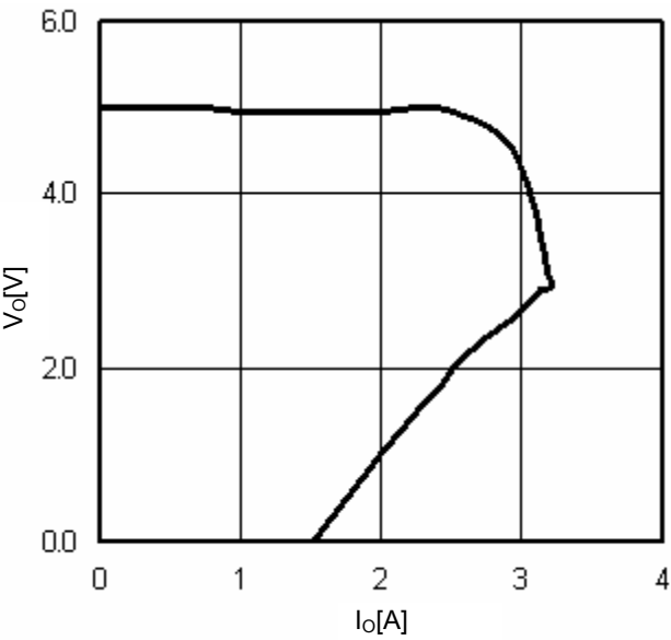
Fig.17 OCP
