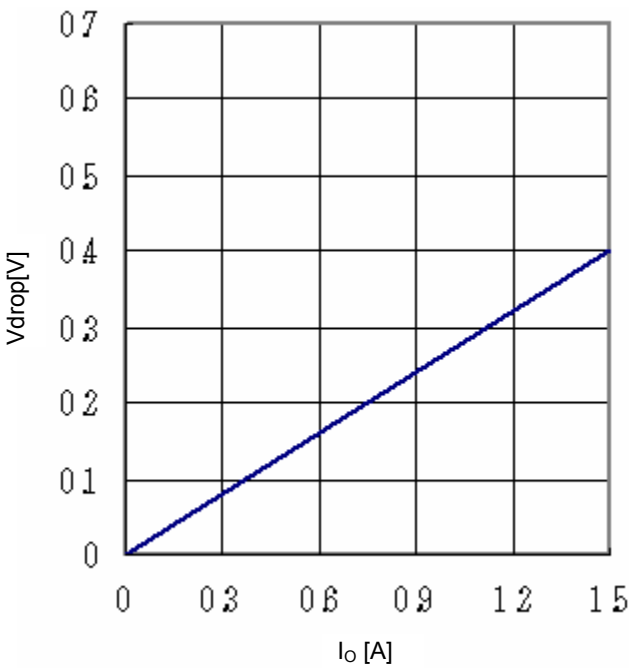
Fig.24 Minimum dropout Voltage 4 ( V_{CC}=8V 、 T_a=25^\circ C )
