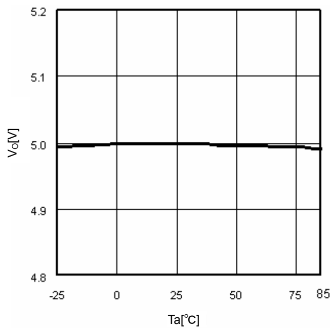
Fig.9 T_a-V_O ( I_o=0mA )
