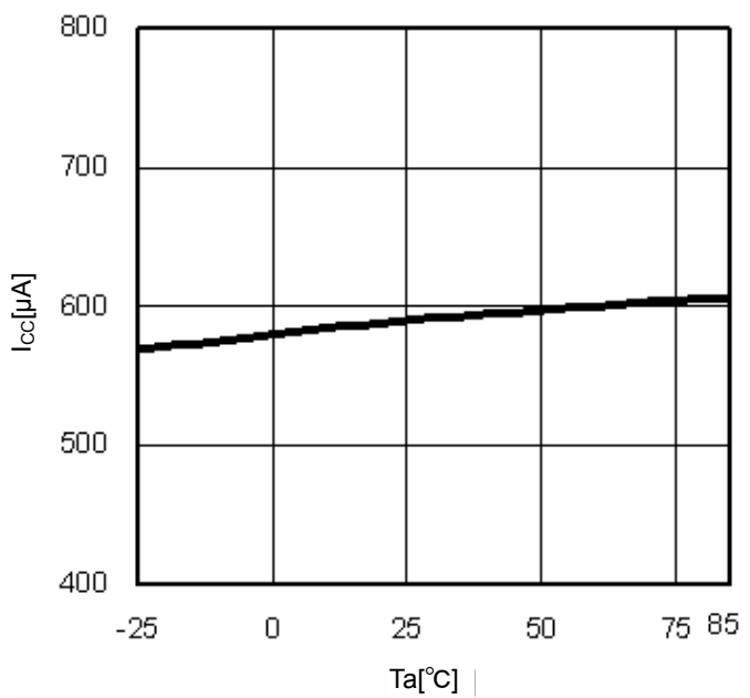
Fig.10 Ta-I CC
