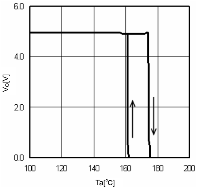
Fig.16 TSD ( I_O=0mA )
