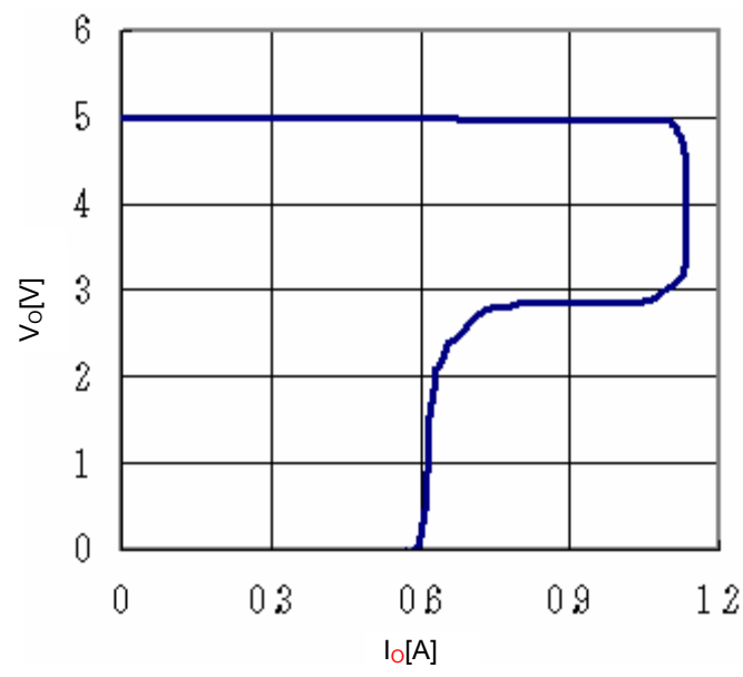
Fig.17 OCP
