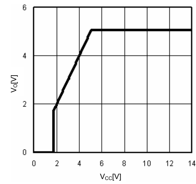
Fig.15 V_{CC}-V_O ( I_O=0mA )
