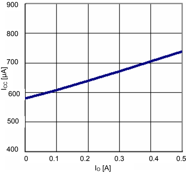
Fig.20 I_o - I_{cc}
