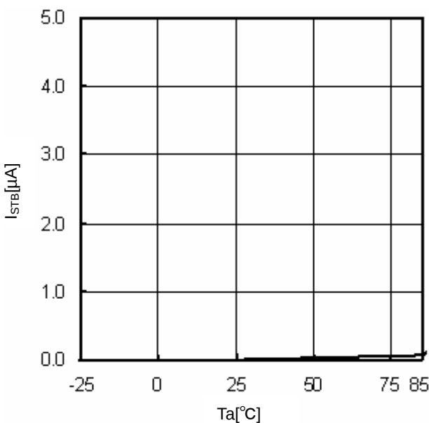
Fig.12 T_a - I_{STB} ( V_{EN}=0\text{V} )
