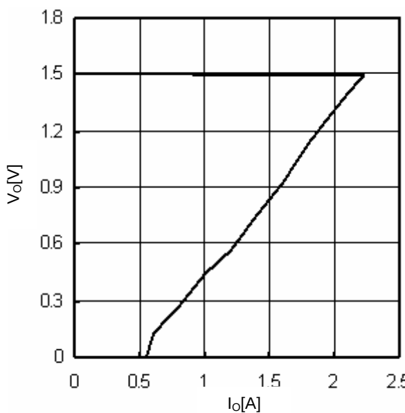
Fig.29 OCP ( V_{cc}=3.3V , V_o=1.5V )
