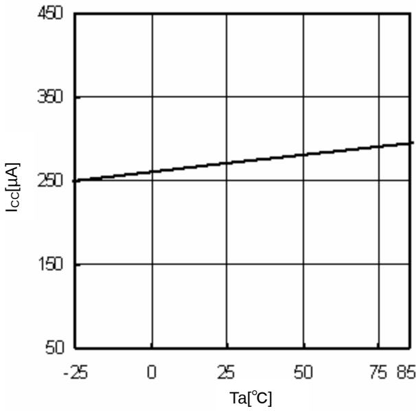
Fig.11 T_a - I_{CC}
