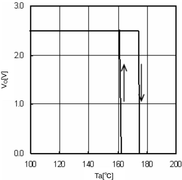
Fig.21 TSD ( I_o=0A )
