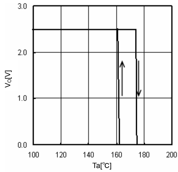
Fig.16 TSD ( I_O=0mA )
