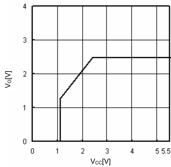
Fig.15 V_{CC}-V_O ( I_O=0mA )
