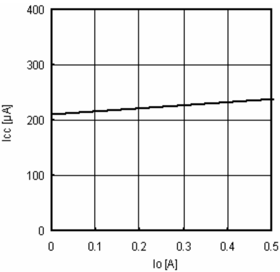
Fig.20 I_o - I_{cc}
