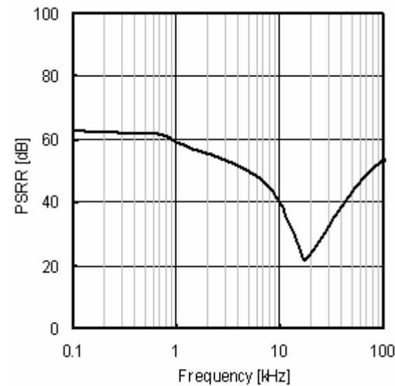
Fig.21 PSRR( I_o=0 mA)
