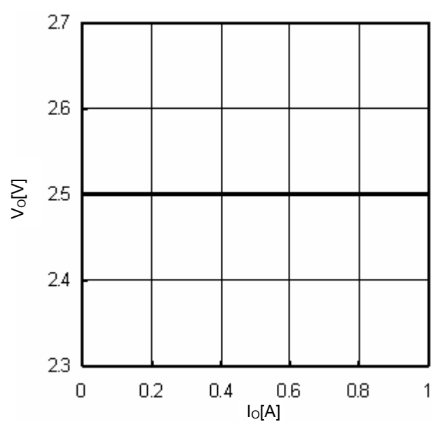
Fig.13 I_O - V_O
