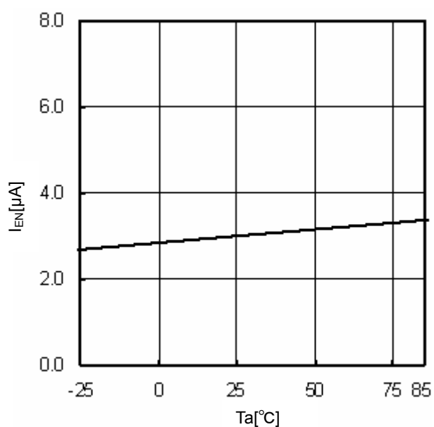
Fig.12 T_a - I_{EN}
