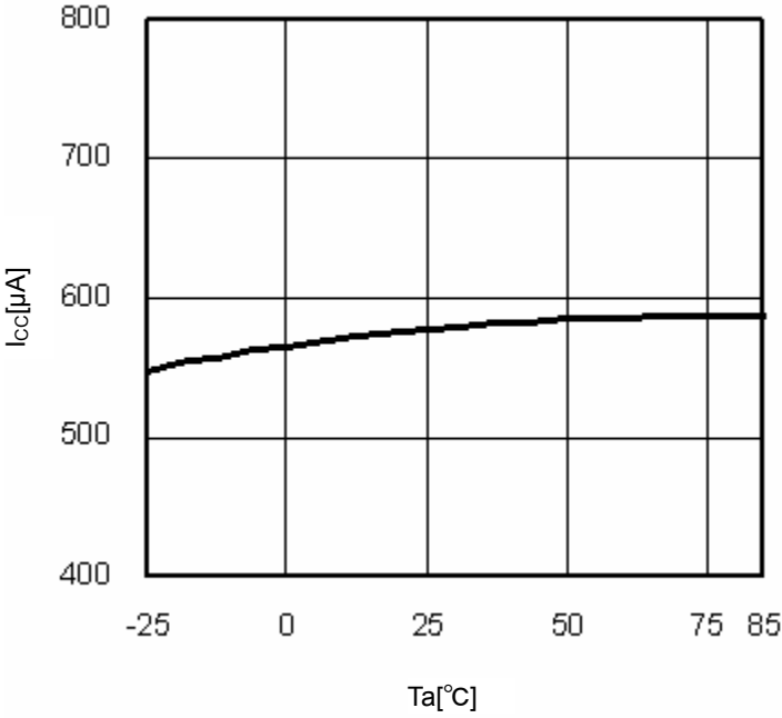
Fig.10 T_a-I_{cc}
