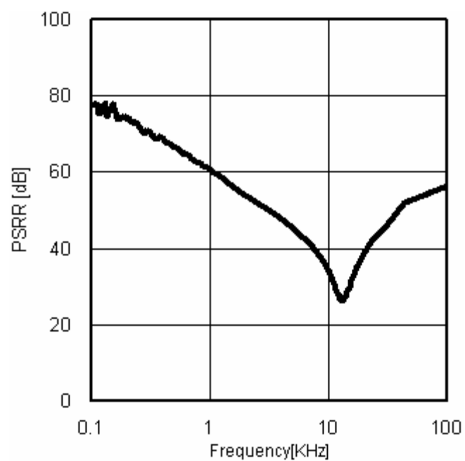
Fig.21 PSRR( I_o=0\text{mA} )
