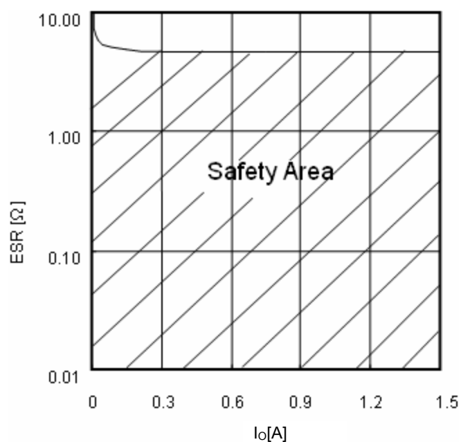
Fig.19 ESR condenser
