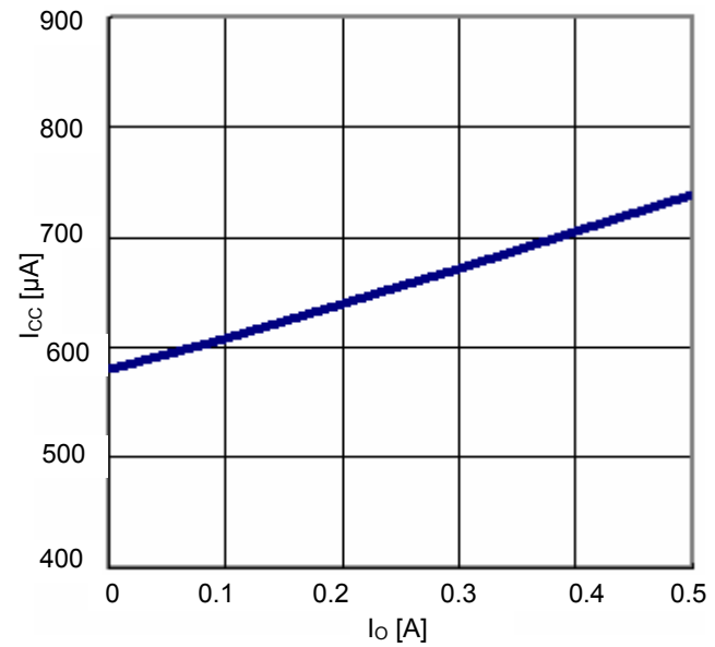
Fig.20 I_o - I_{cc}
