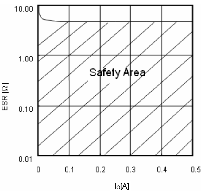
Fig.19 ESR condenser
