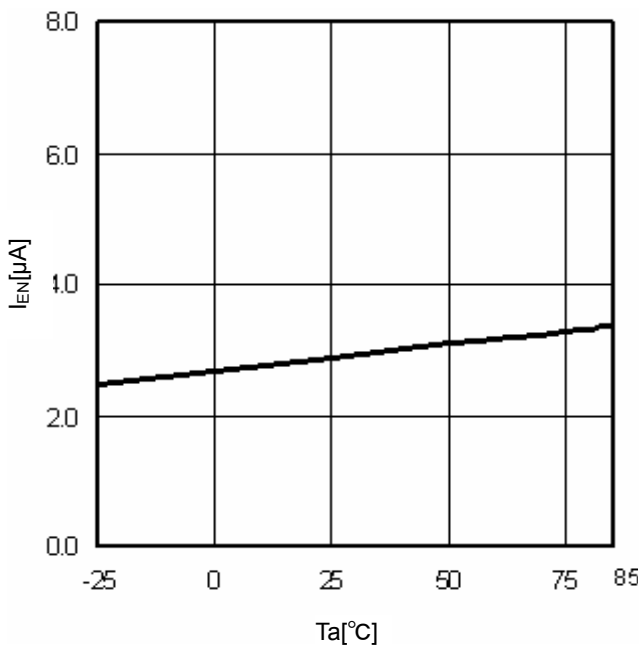
Fig.12 T_a - I_{EN}
