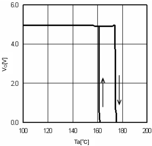
Fig.16 TSD ( I_O=0mA )
