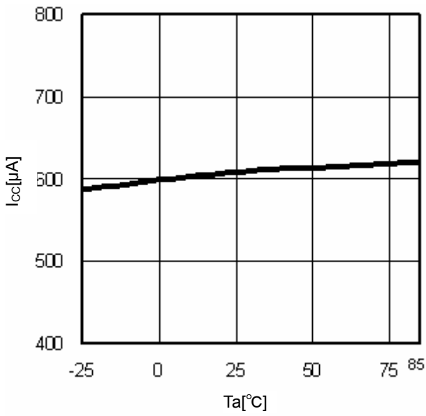
Fig.10 T_a-I_{cc}
