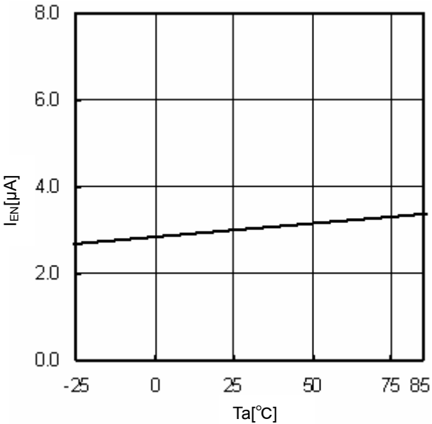
Fig.12 T_a - I_{EN}
