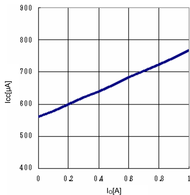
Fig.20 I_o - I_{cc}
