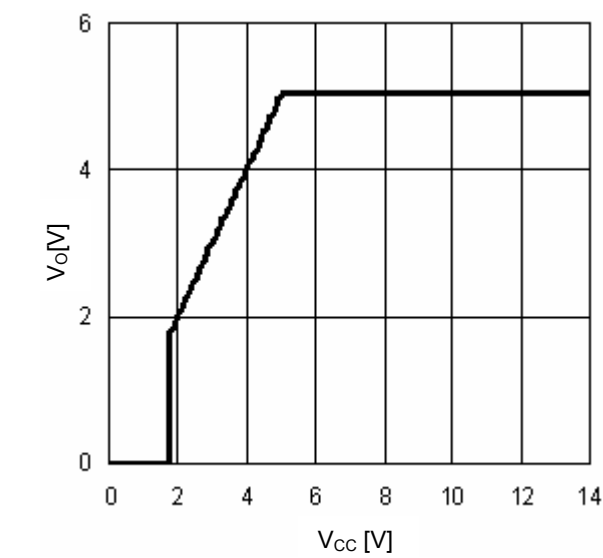
Fig.15 V_{CC}-V_O ( I_O=0mA )
