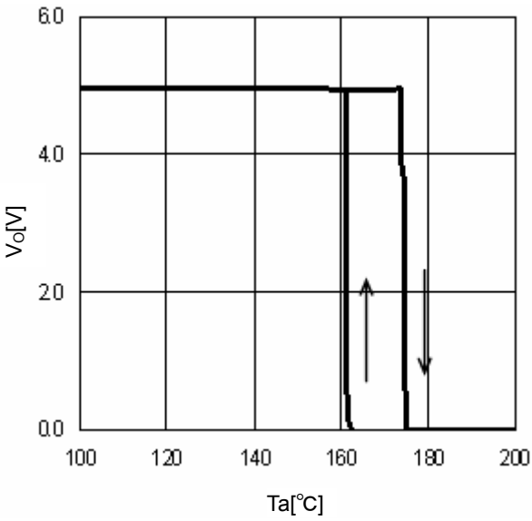
Fig.16 TSD ( I_O=0mA )
