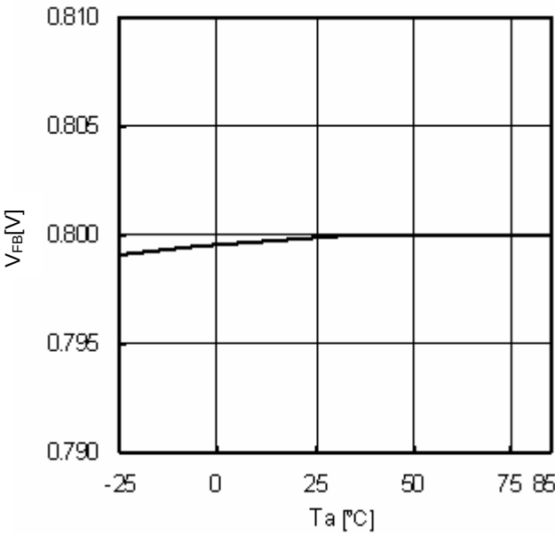
Fig.9 T_a-V_{FB}
