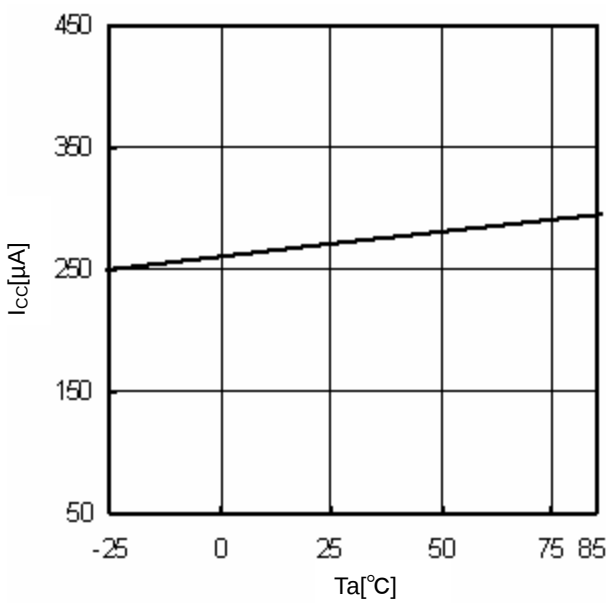
Fig.11 T_a - I_{CC}
