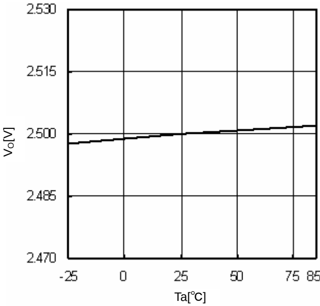
Fig.10 T_a-V_O ( I_o=0A )
