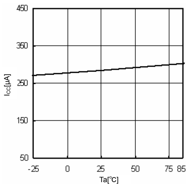
Fig.10 T_a - I_{CC}
