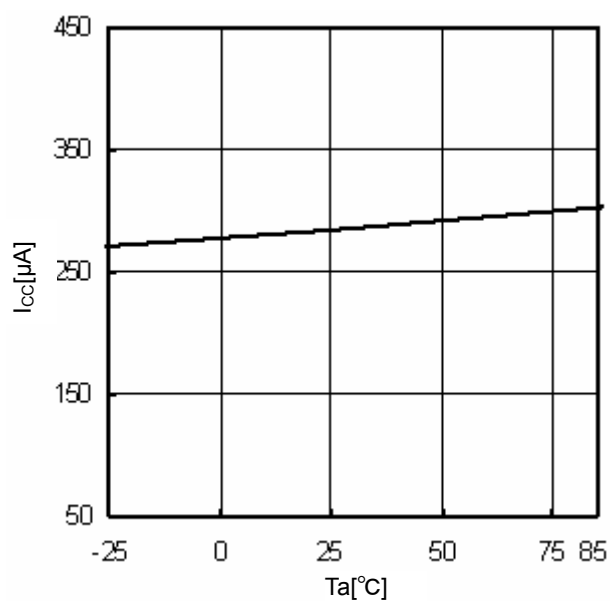
Fig.10 Ta- I_{CC}
