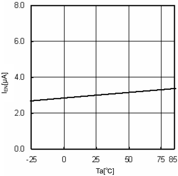
Fig.12 T_a - I_{EN}
