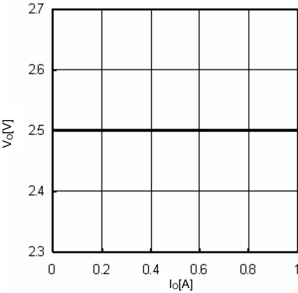
Fig.13 I_O - V_O
