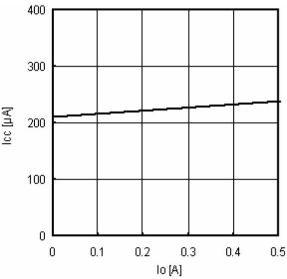
Fig.20 Io-Icc
